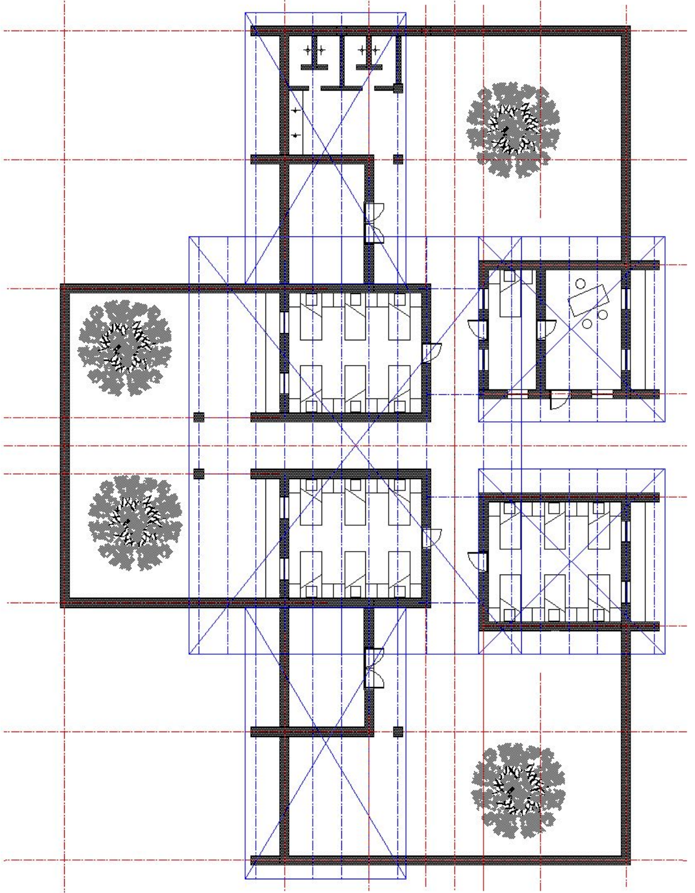
2- Dapelogo : le 1 er module (plan non coté)
